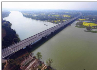
沱江河特大桥
