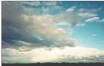
雨层云
