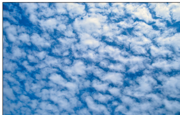
高积云
