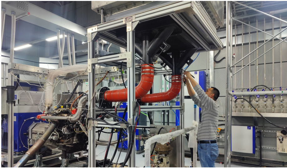
国家环境保护机动车污染控制与模拟重点实验室(成都基地)发动机试验室内,工作人员正在进行设备调试。
