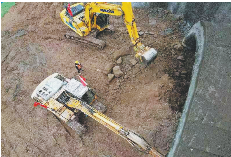
成达万高铁光明隧道口施工现场。
