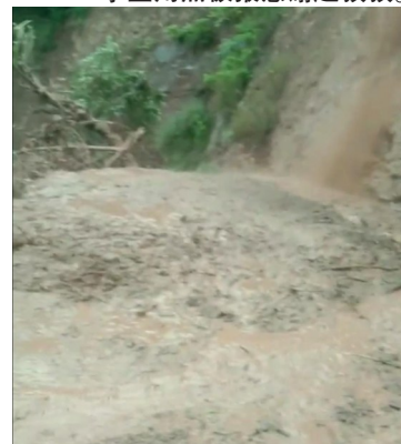
泥石流现场。
